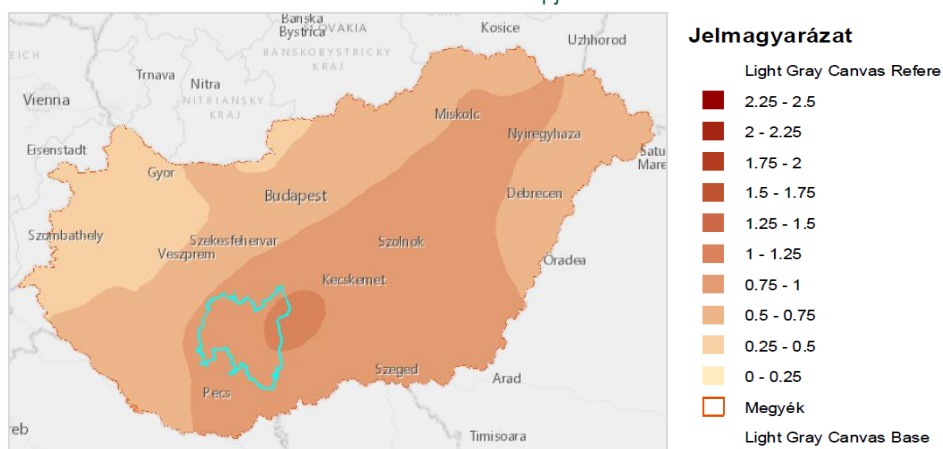
23. ábra A módosított Pálfi-féle aszályindex várható változása a 2021–2050 időszakra az ALADIN-Cilimate klímamodell alapján
